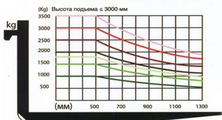
График грузоподъемности
