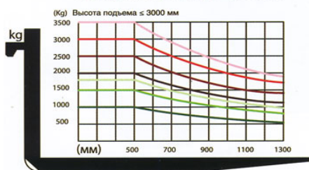
График грузоподъемности
