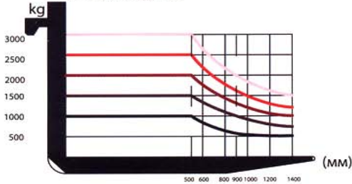
График грузоподъемности
